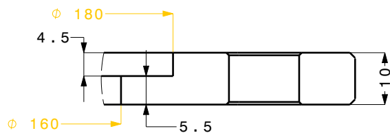
Detail K Scale: 1:1
