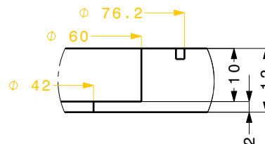
Detail M Scale: 1:1
